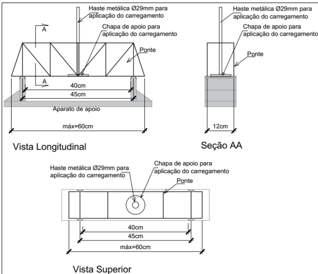
Figura 4: Esquema de apoio e carregamento da ponte.
